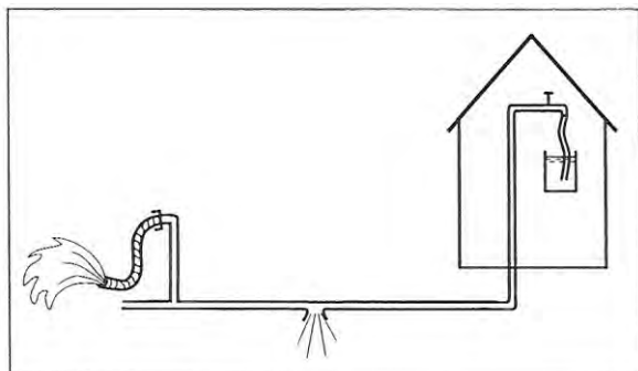
Figur 2.6 Tilbageløb ved undertryk i forsyningsledningen
